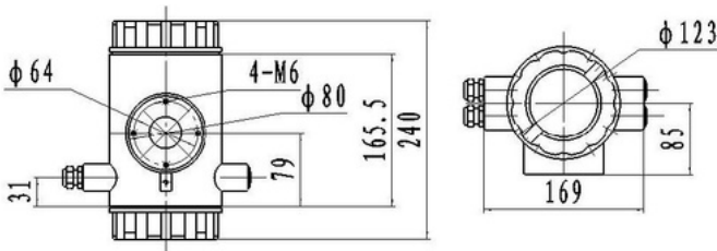
Fig.1 Dimensional do invólucro circular integrado
