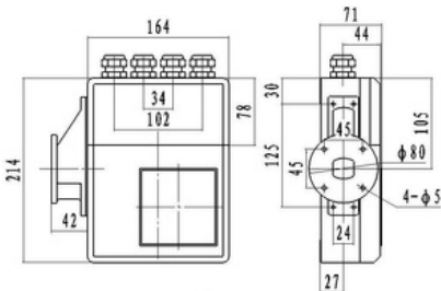
Fig.2 Dimensional do invólucro retangular remoto
